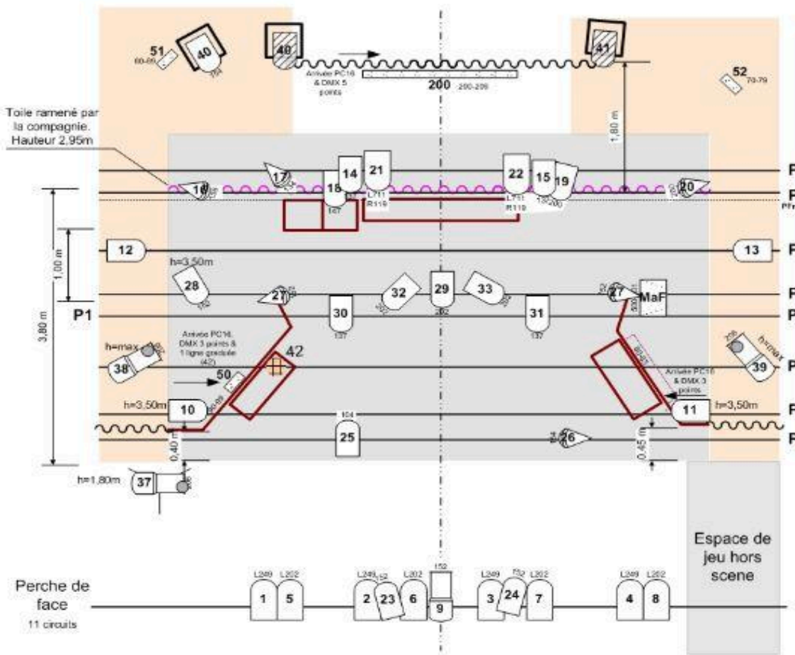
VISUEL DU PLAN DE CONTRE (10) (14) (22) (29) (32) (33) (39) VUE DE FACE
